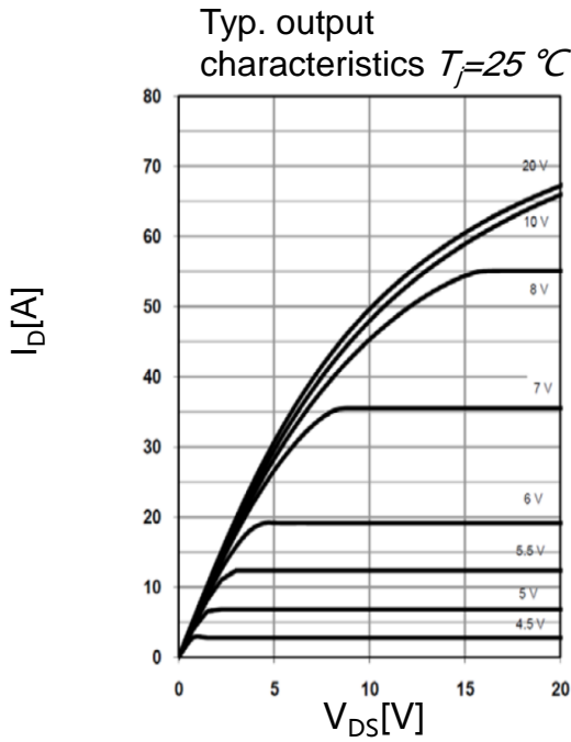
I_D=f(V_{DS}); T_j=25^\circ\text{C} ; parameter: V_{GS}
