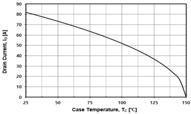
Fig. 9 I_D - T_C
