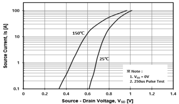
Fig. 4 I_S - V_{SD}
