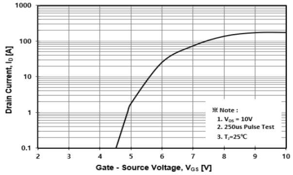
Fig. 2 I_D - V_{GS}
