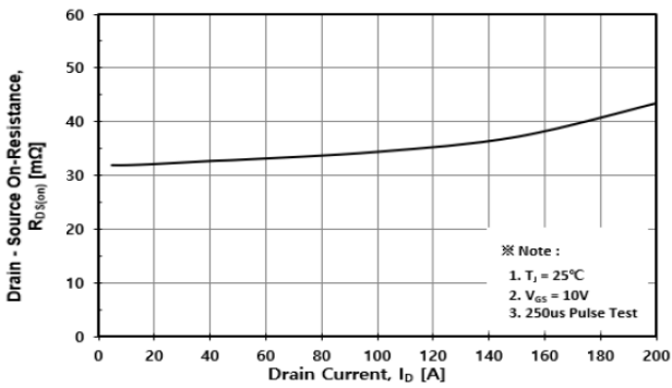
Fig. 3 R_{DS(ON)} - I_D
